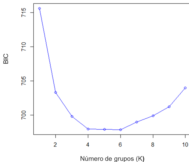
Figura 4. Número de agrupamentos encontrados no DAPC para os 169 isolados de Corynespora cassiicola conforme o critério de inferência bayesiana (BIC). O menor valor de BIC representa o melhor número de grupos (K=4).
