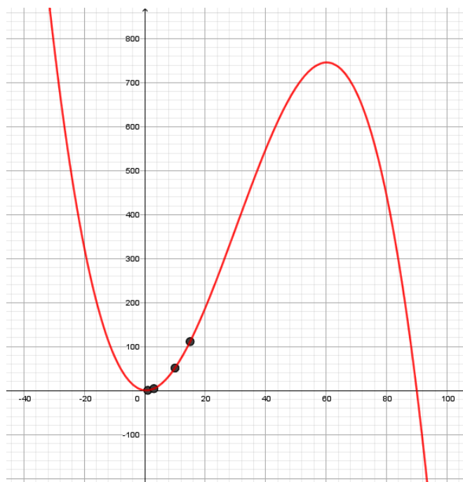
Figura 4.14: Gráfico de X(t) estendido.
