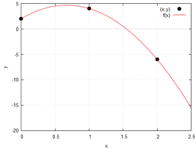
Figura 2.3: Função interpoladora f(x) = -6x^2 + 8x + 2 .
