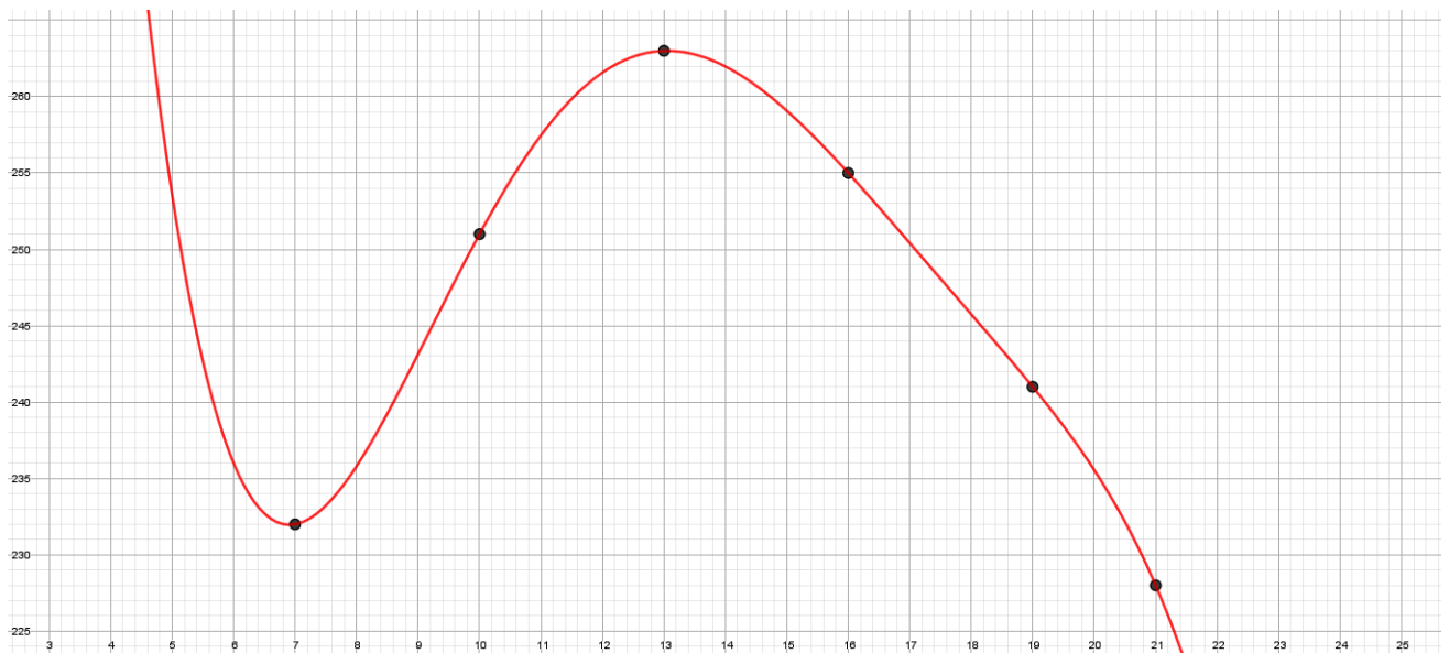
Figura 4.16: Gráfico da função interpoladora g(x) .
