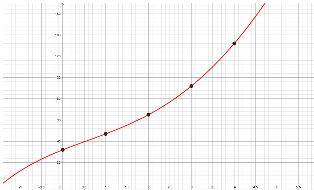
Figura 4.17: Gráfico do polinômio interpolador y(x) .
