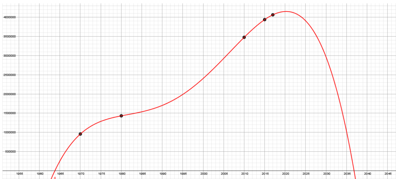
Figura 4.13: Função polinomial interpoladora p(x) .
