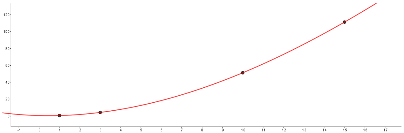
Figura 4.15: Gráfico de X(t) entre 1 e 15 ut.
