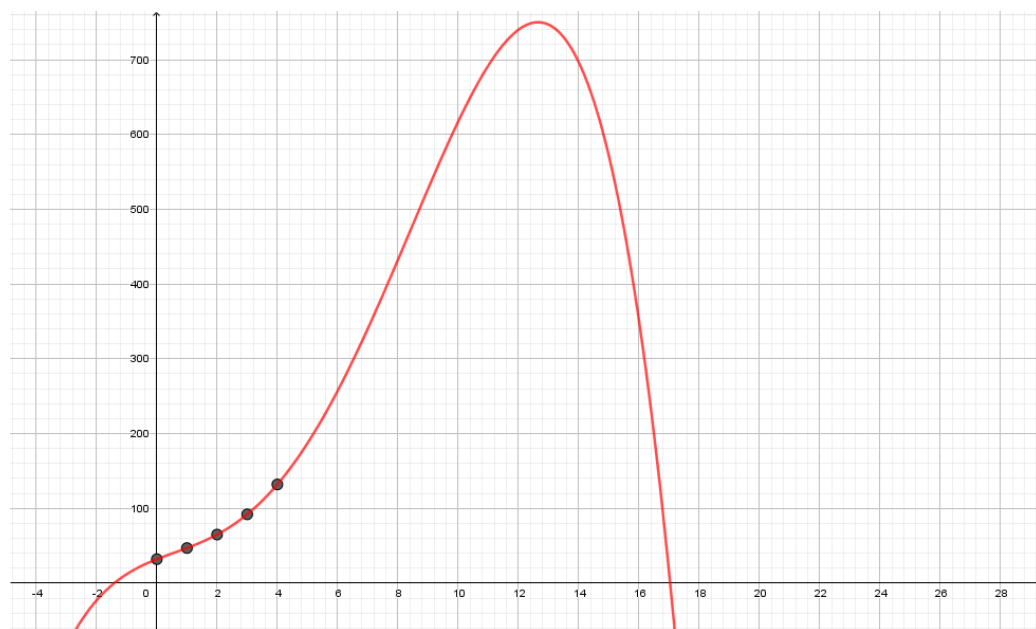
Figura 4.18: Gráfico do polinômio interpolador y(x) expandido.
